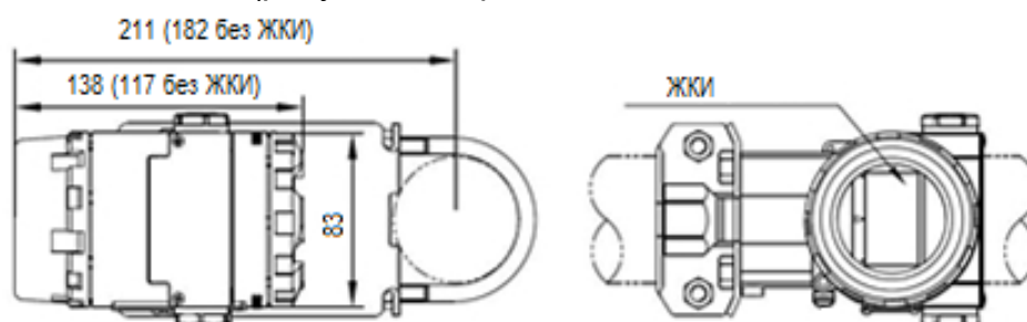
Рисунок 6 – Монтаж на горизонтальный импульсный трубопровод датчиков штырьного исполнения
